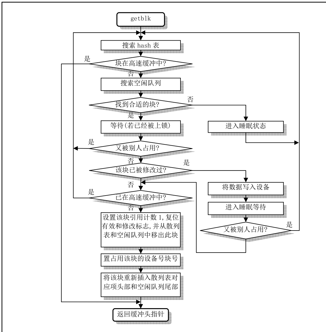
图 12-20 getblk() 函数执行流程图
