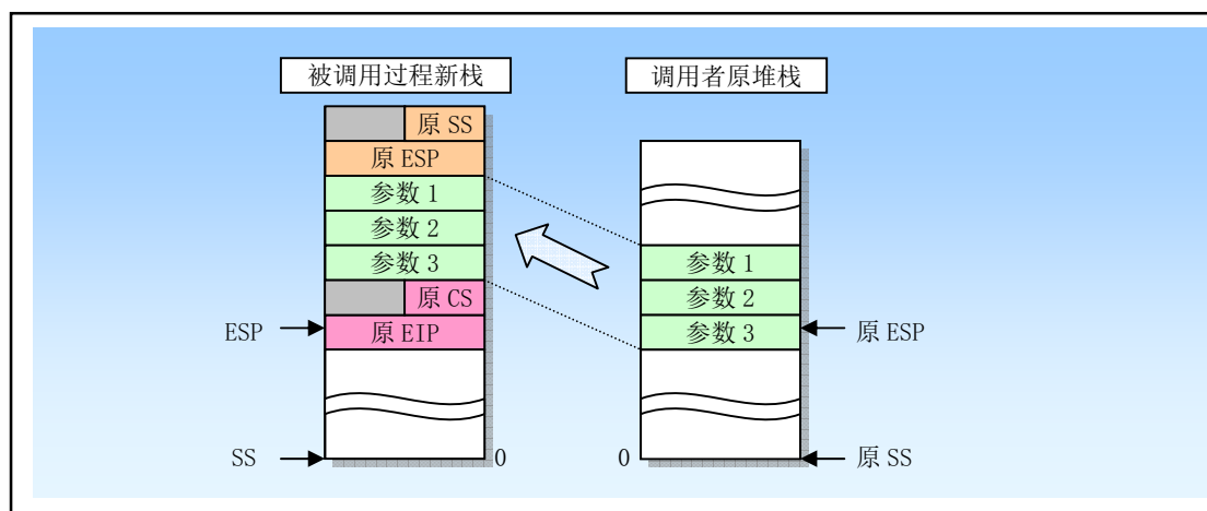
图 4-25 不同特权级之间调用时的栈切换
