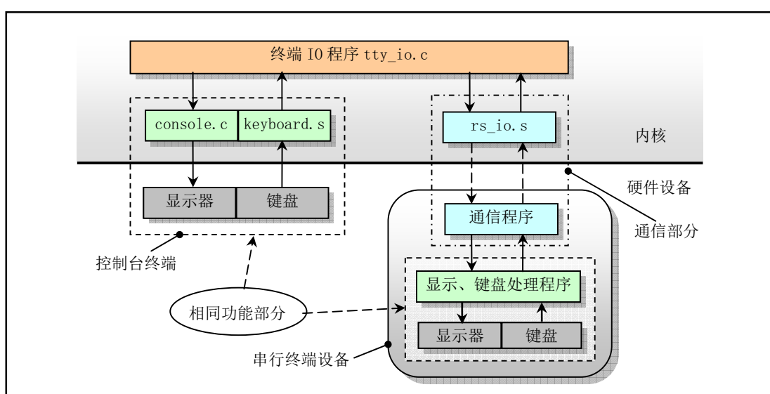
图 10-3 控制台终端与串行终端设备示意图
