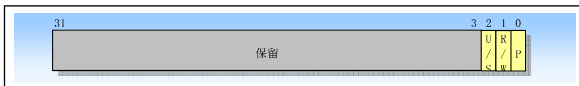
图 4-32 页面故障错误码格式
