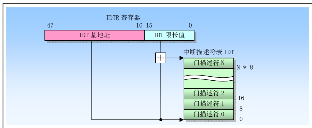
图 4-26 中断描述符表 IDT 和寄存器 IDTR
