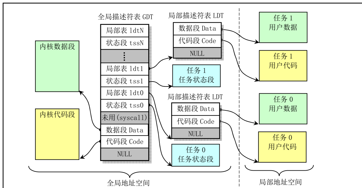
图 5-8 Linux 系统中虚拟地址空间分配图
