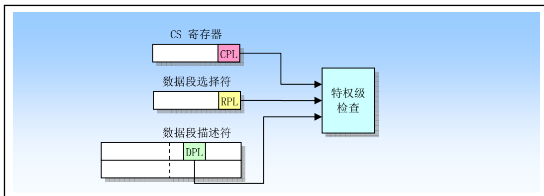
图 4-20 访问数据段时的特权级检查
