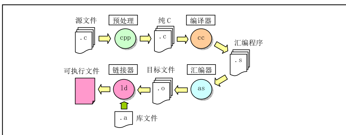
图 3-3 C 程序编译过程
