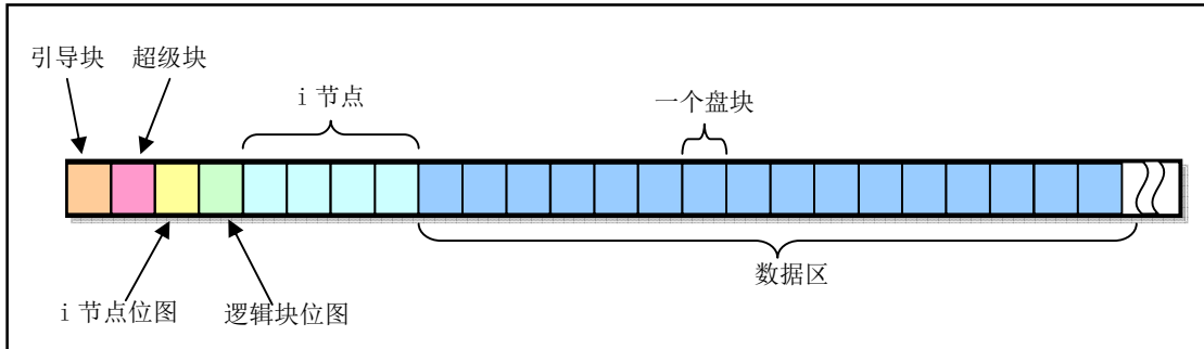
图 12-1 建有 MINIX 文件系统的 360K 软盘中文件系统各部分的布局示意图
