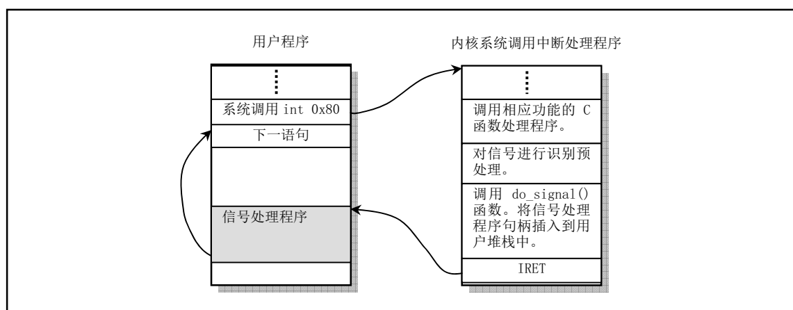
图 8-10 信号处理程序的调用方式。
