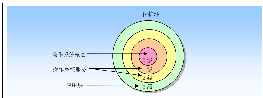
图 4-19 处理器特权级示意图
